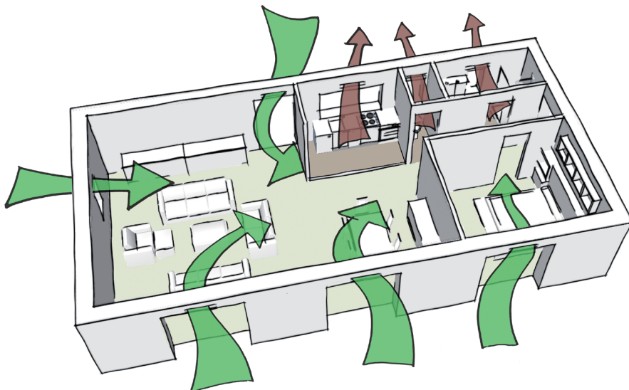
Le principe de la ventilation est d'apporter de l'air neuf dans les pièces de vie (salon, chambres) et d'extraire l'air vicié depuis les pièces « humides » (cuisine, sanitaires).
